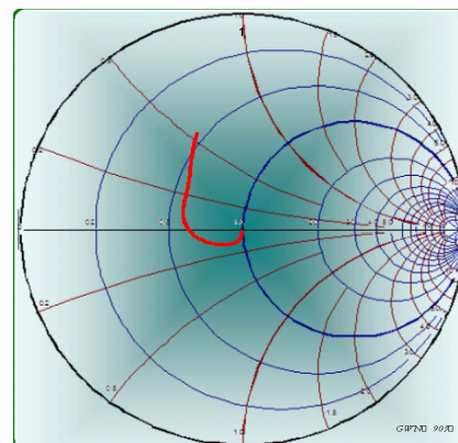
Figure4: B2504-C3, Into 50Ω
